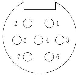
A. 7-Core Input Terminal
