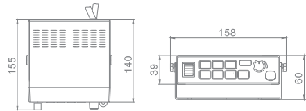
CJB-10002 | 100W Siren
